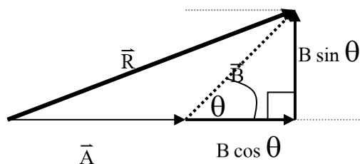
รูป 2. เวกเตอร์ลัพธ์ \vec{R} หาได้โดยใช้กฎพีทาгорัส
