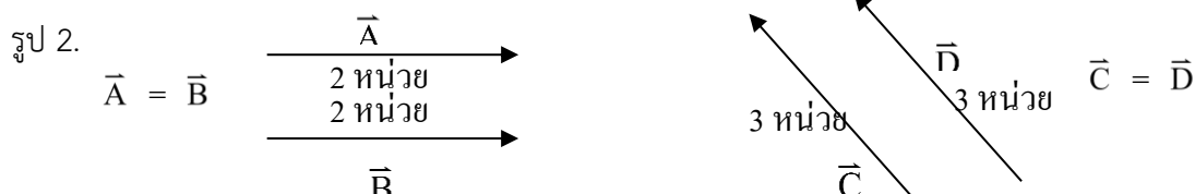
รูป 2. แสดงเวกเตอร์ที่เท่ากัน
