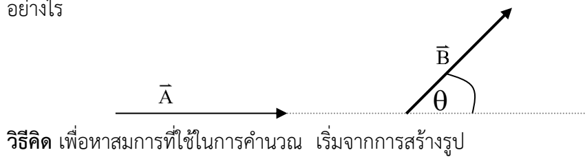
รูป 1. แยก \vec{B} เพื่อหาขนาดเวกเตอร์ลัพธ์ \vec{R}
